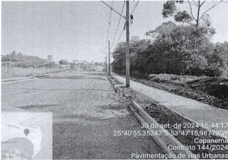
Figura 04- Rua Cariris, serviços de urbanização, e base.
