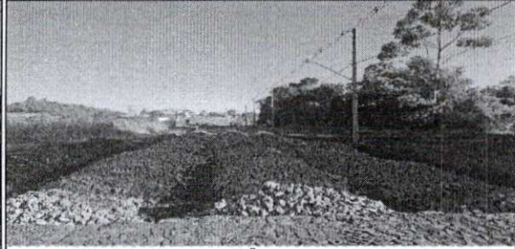
6 | LIMPEZA, REGULARIZAÇÃO SUBLEITO, MATERIAL SUB-BASE, RUA CARIRIS
