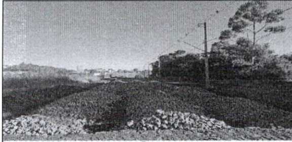
5 | LIMPEZA, REGULARIZAÇÃO SUBLEITO, MATERIAL SUB-BASE, RUA CARIRIS
